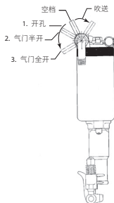
图1.(Dwg. 16578304) 操作杆定位
