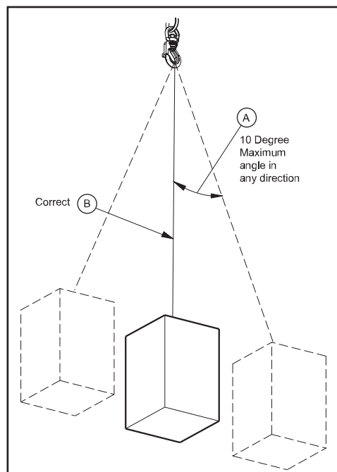
(Dwg. MHP2649)
